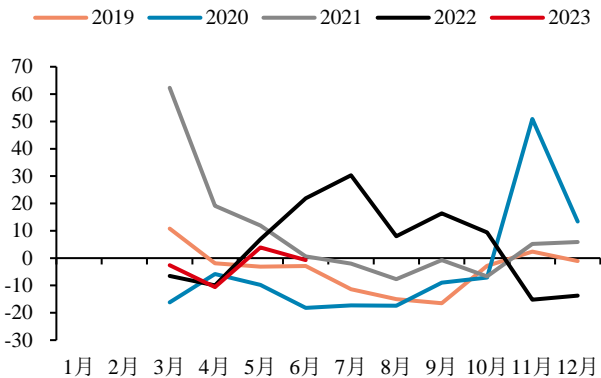
图 67: 工业锅炉产量当月同比 | 单位: %
