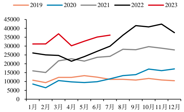
图 34: 中国硫酸镍金属产量 | 单位: 镍吨
