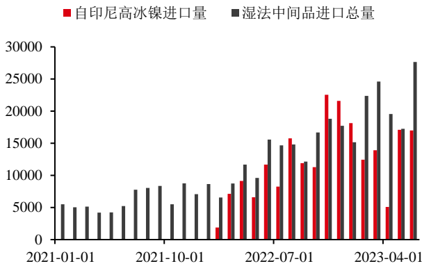
图 13: 中国主要镍中间品进口量 | 单位: 镍吨
