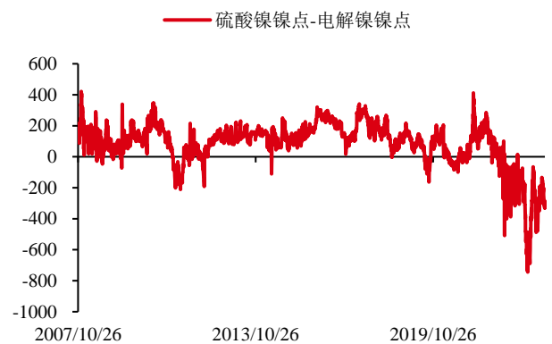
图 32: 中国精炼镍与硫酸镍价差 | 单位: 元/镍点
