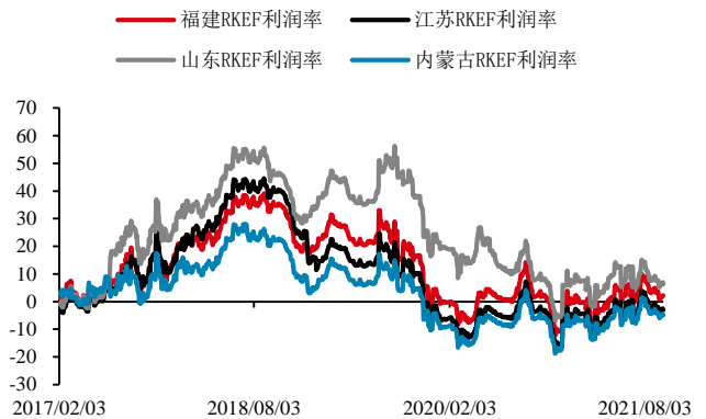
图 14: 中国高镍铁 RKEF 利润率 单位: %
