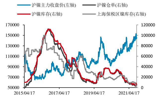
图 10: 中国沪镍与保税区库存 单位: 元/吨、吨
