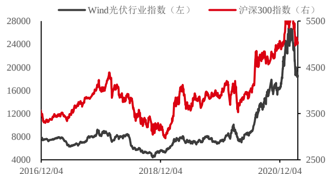
图 18: 申万光伏行业板块指数 单位: 点
