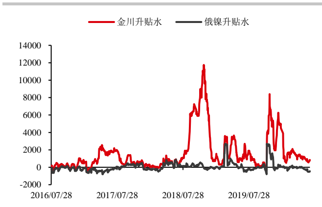
图 2: SMM 电解镍升贴水 单位: 元/吨
