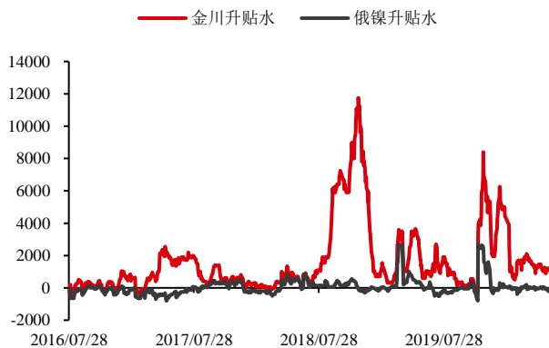
图 2: SMM 电解镍升贴水 单位: 元/吨
