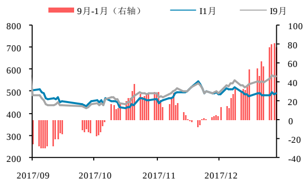
图 5：铁矿石 9 月-1 月
