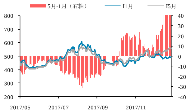
图 6：铁矿石 5 月-1 月
