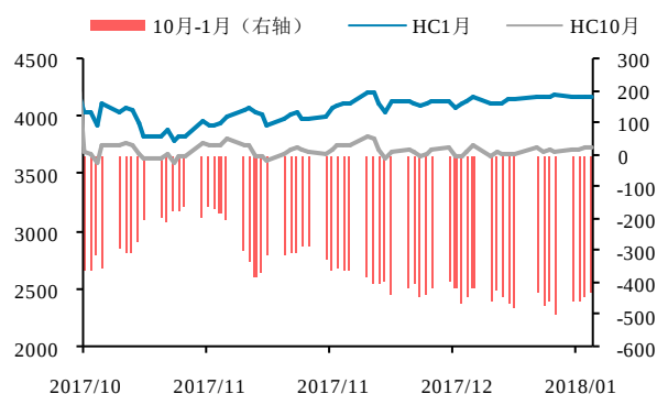
图 3：热轧 10 月-1 月
