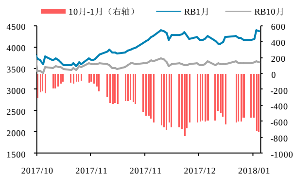
图 1：螺纹 10 月-1 月
