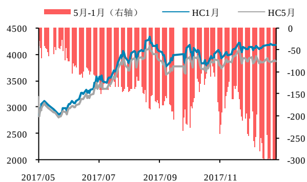
图 4：热轧 5 月-1 月
