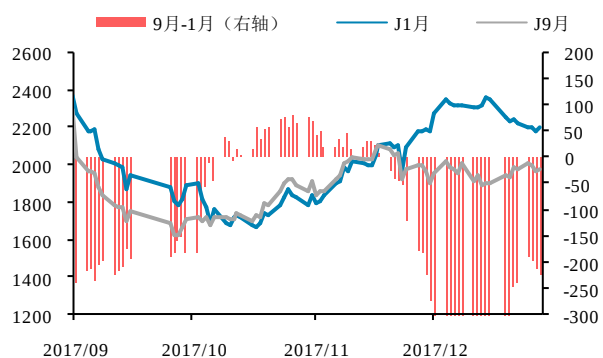
图 7：焦炭 9 月-1 月
