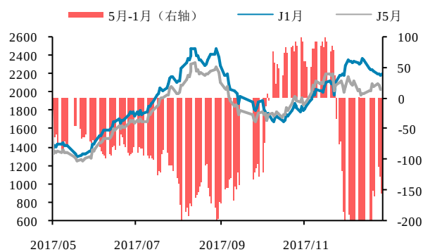
图 8：焦炭 5 月-1 月
