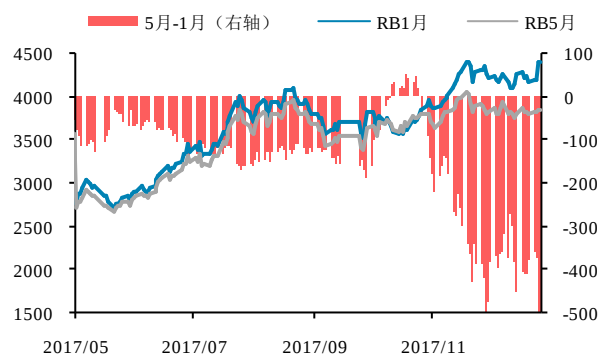
图 2：螺纹 5 月-1 月
